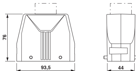
尺寸图
