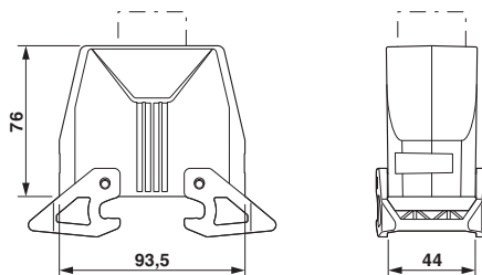
尺寸图
