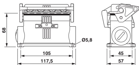
尺寸图
