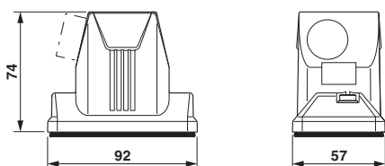
尺寸图
