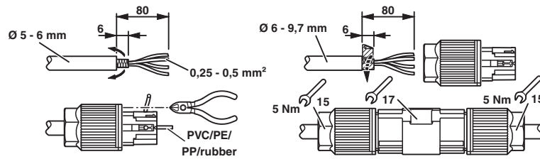
功能图
