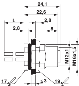
尺寸图
