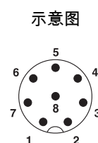
M8针式连接器引脚分配, 8芯, 插头侧视图
