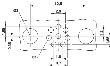
钻孔图
