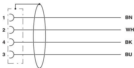
电路图
