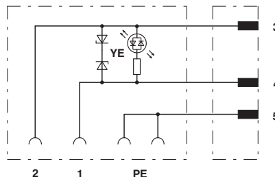
M12 针式/阀插头的引脚分配
