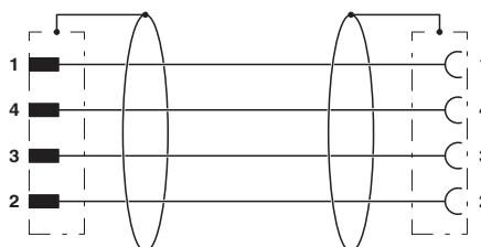
电路图
