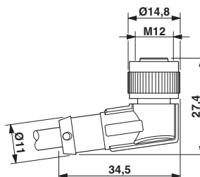
尺寸图
