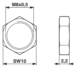
尺寸图
