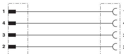
电路图
