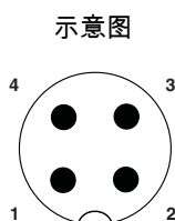
M12针式连接器引脚分配，4芯，A编码，插头侧视图
