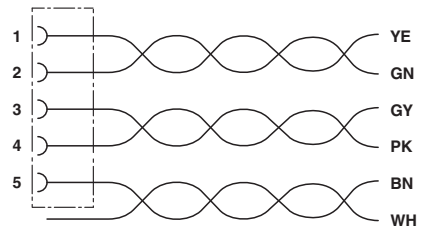
电路图
