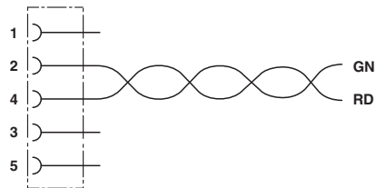
电路图
