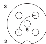
M12孔式连接器引脚分配, 3芯, 桥接, PE, A编码, 插座侧视图
