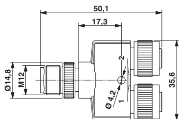
M12 x 1连接器, Y型分配器, 内径21mm
