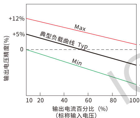
误差包络曲线图 3.3Vdc输出
