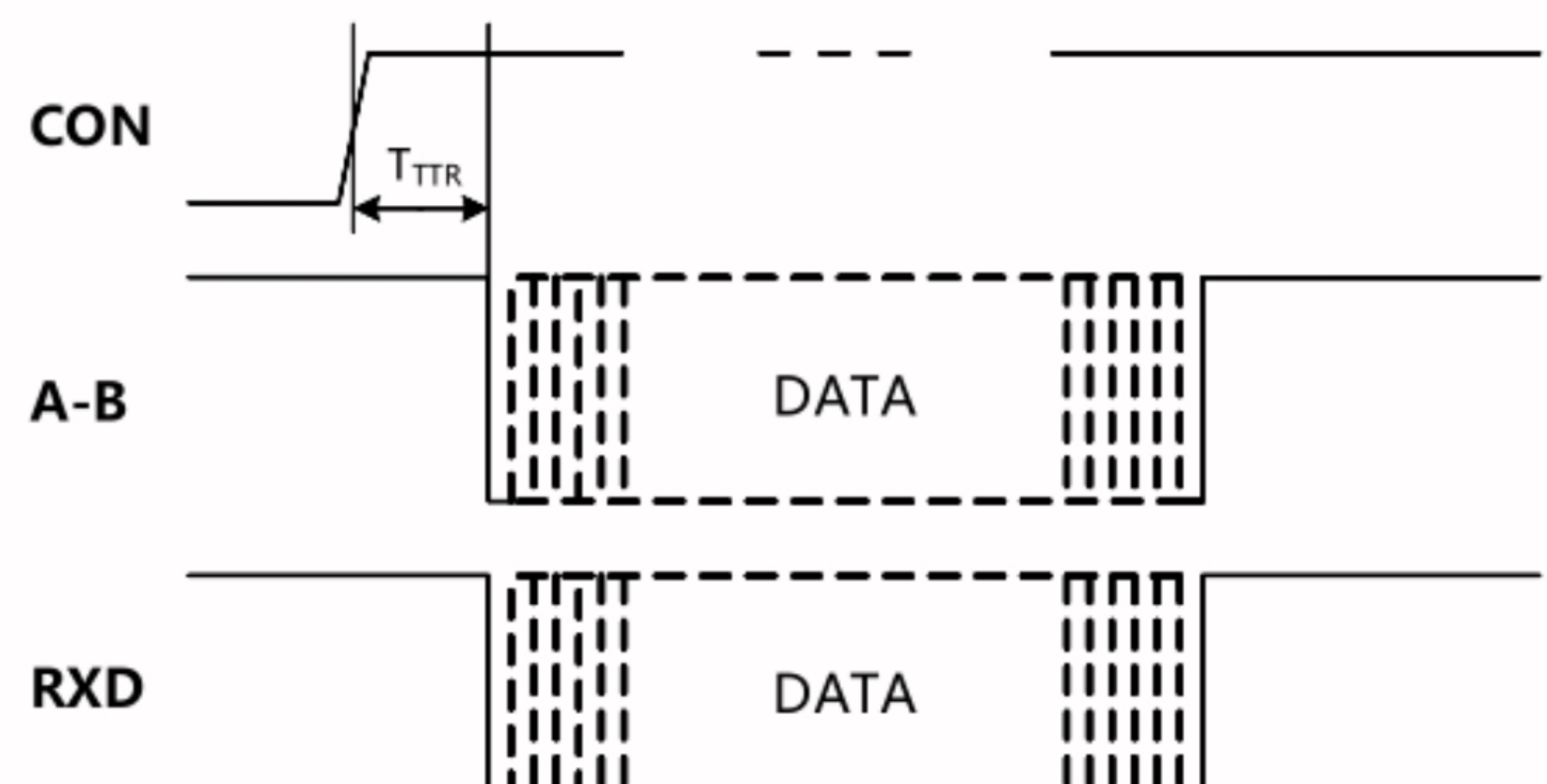
图2. RSM(3)485PCT模块数据接收时序图
