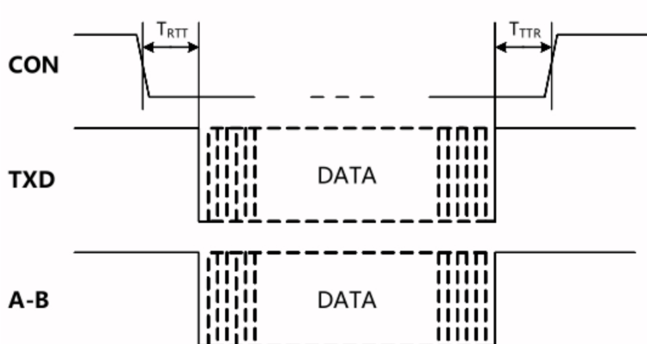
图1. RSM(3)485PCT模块数据发送时序图
