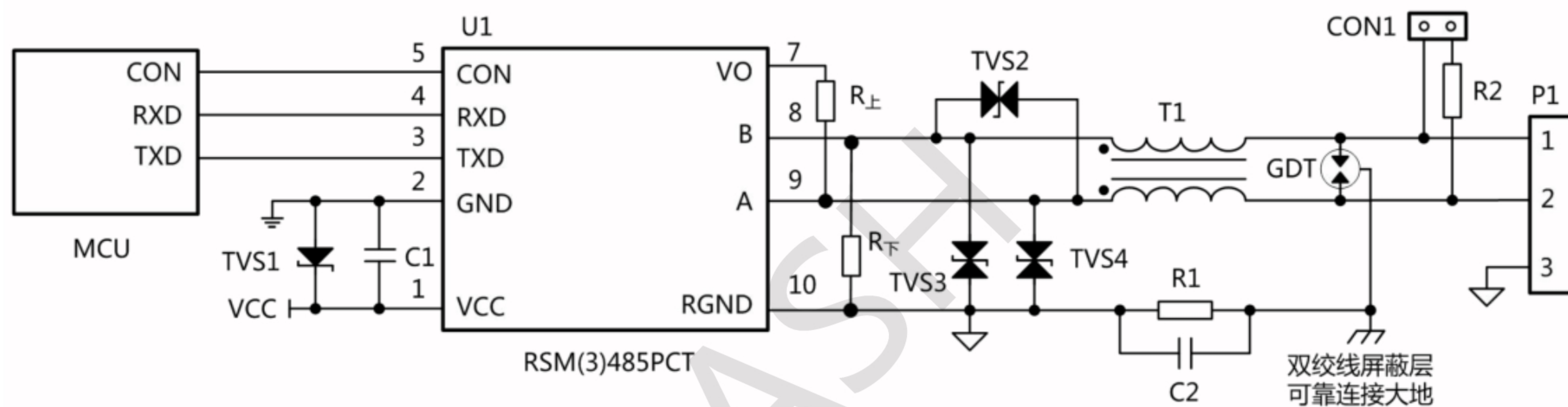
图5. EMC推荐电路
